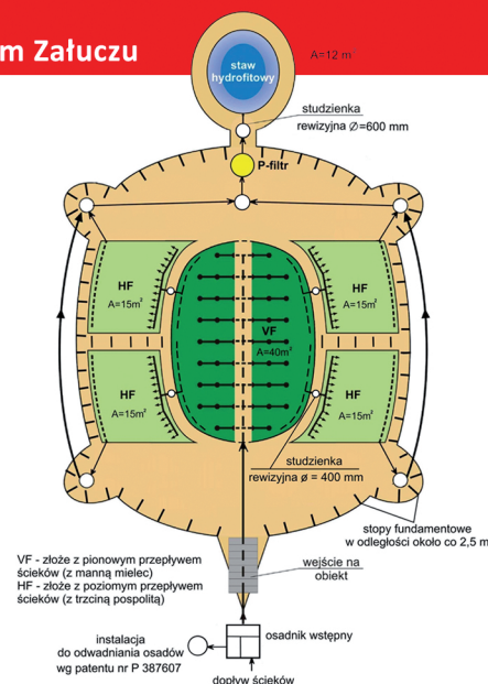
Załącznik 2. Schemat techniczny hybrydowej hydrofitowej oczyszczalni ścieków dla Ośrodka Dydaktyczno-Muzealnego Poleskiego Parku Narodowego w Starym Załuczu
