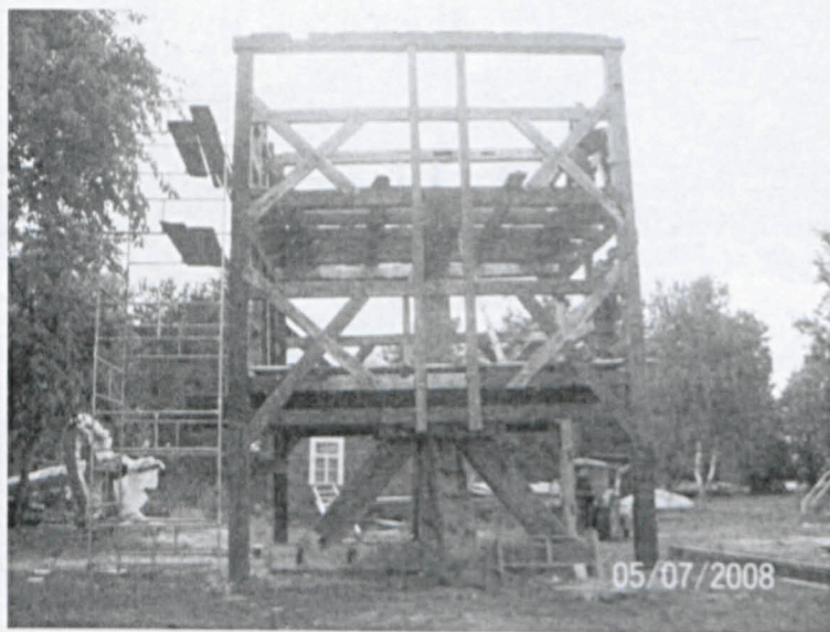
Fot. nr 119. Konstrukcja nośna wiatraka wykonana przez cieślę Jana Baja
