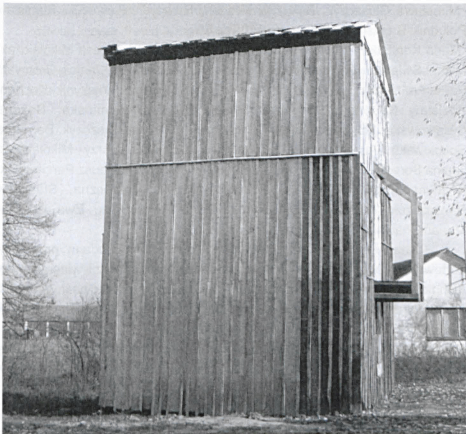
Fot. nr 120. Konstrukcja nośna odeskowana i zabezpieczona przez seniorów
