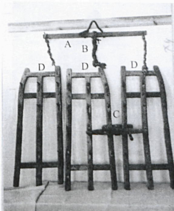
Fot. nr 75. Brony ( II poł. XIX w.) A. Orczyca, B. Wiązadła z korzenia, C. Łącznik D. Komplet bron-trojaki
