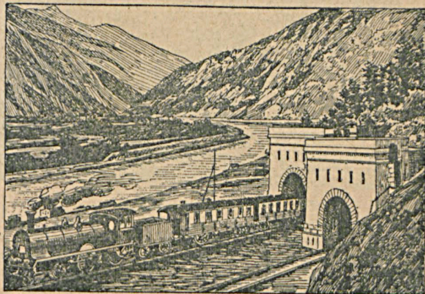
Tunel symplonński.
