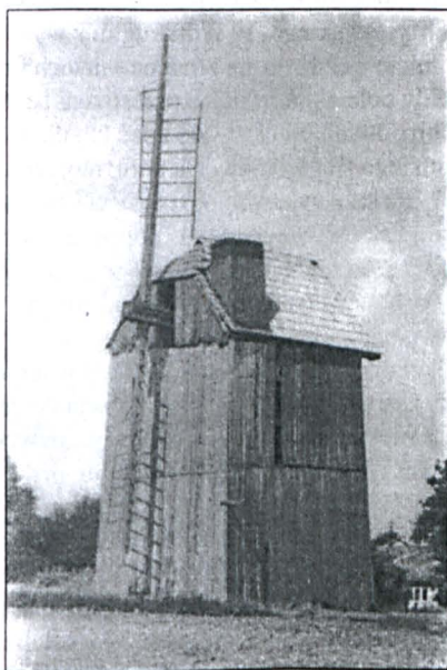
Wiatrak (koźlak) Stanisława Nazarewskiego. Fot. autora (1984 r.).
