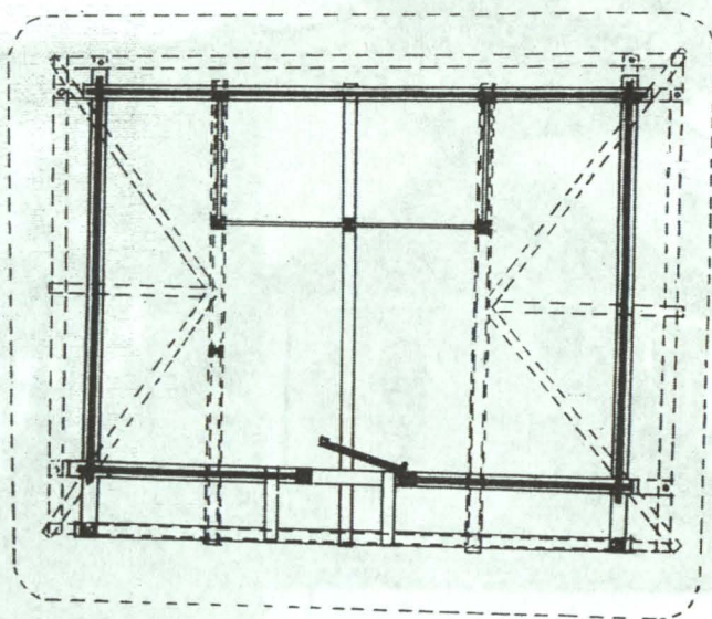
Kornica, plan jednokomorowego spichrza podcieniowego z XIX w.
