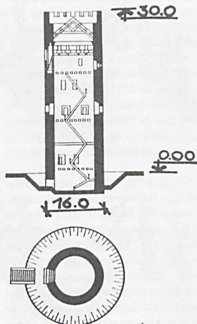
План і поперечний розріз Кам'янецького стовпа
