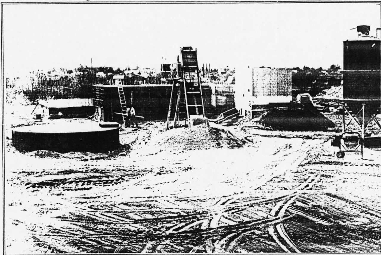
Ocyszczalnia ścieków
