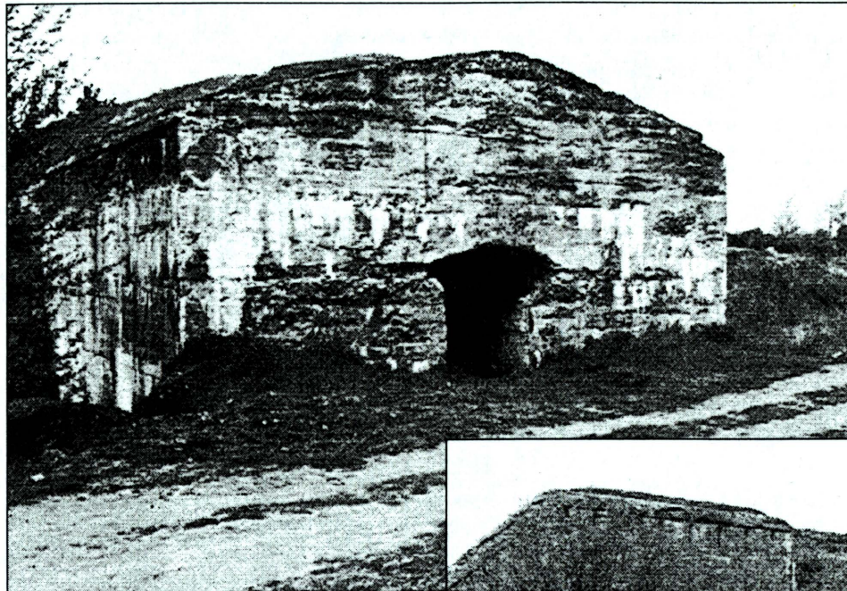
Fort LEBIEDZIEW - poterna osiowa, urywająca się równym segmentem po wysadzeniu kapaniery. Zwraca uwagę grubość betonu do 5m!
