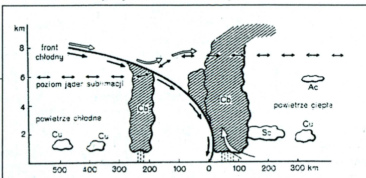
Schemat chmur związanych z frontem chłodnym.
