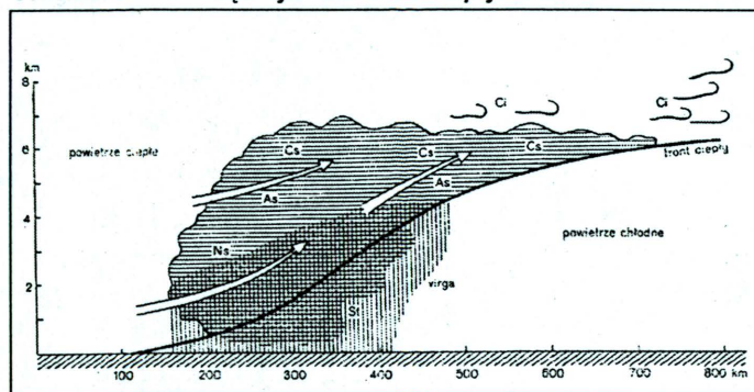
Schemat chmur związanych z frontem ciepłym
