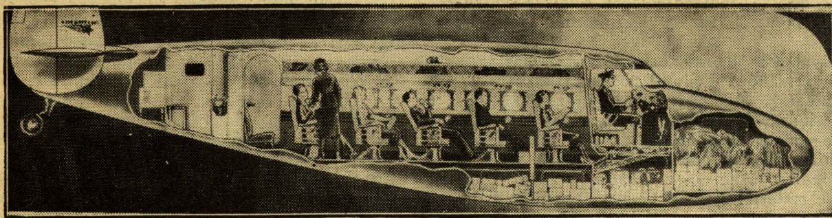
Polskie Linie Lotnicze nabyły dla polskiej komunikacji powietrznej nowego typu samoloty pasażerskie. Wnętrze nowego samolotu — w przekroju.
