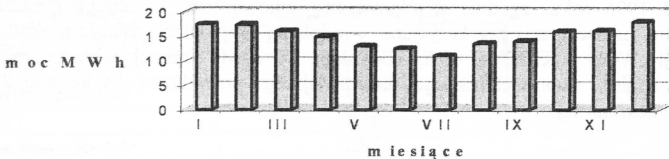
Wykres 6. Miesięczne szczytowe obciążenie (mocą czynną) głównych punktów zasilania Białej Podlaskiej w 1999 r.
