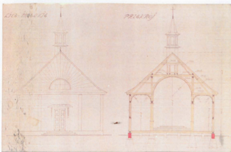
Projekt drewnianego kościoła
