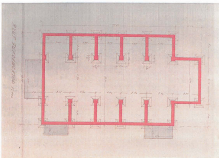
Projekt drewnianego kościoła – rzut fundamentów
