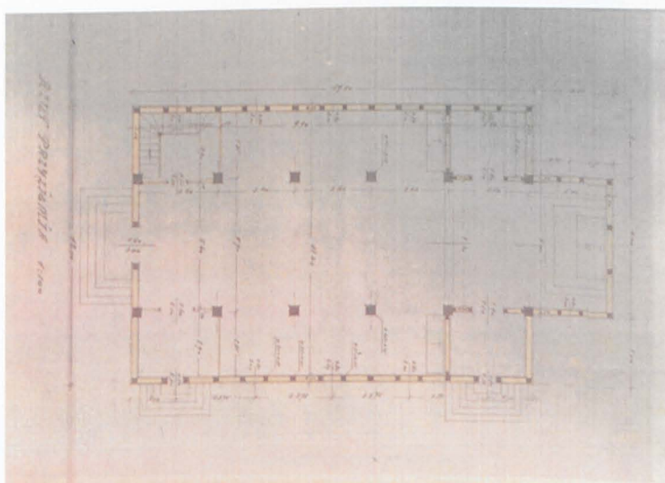
Projekt drewnianego kościoła – rzut przyziemia
