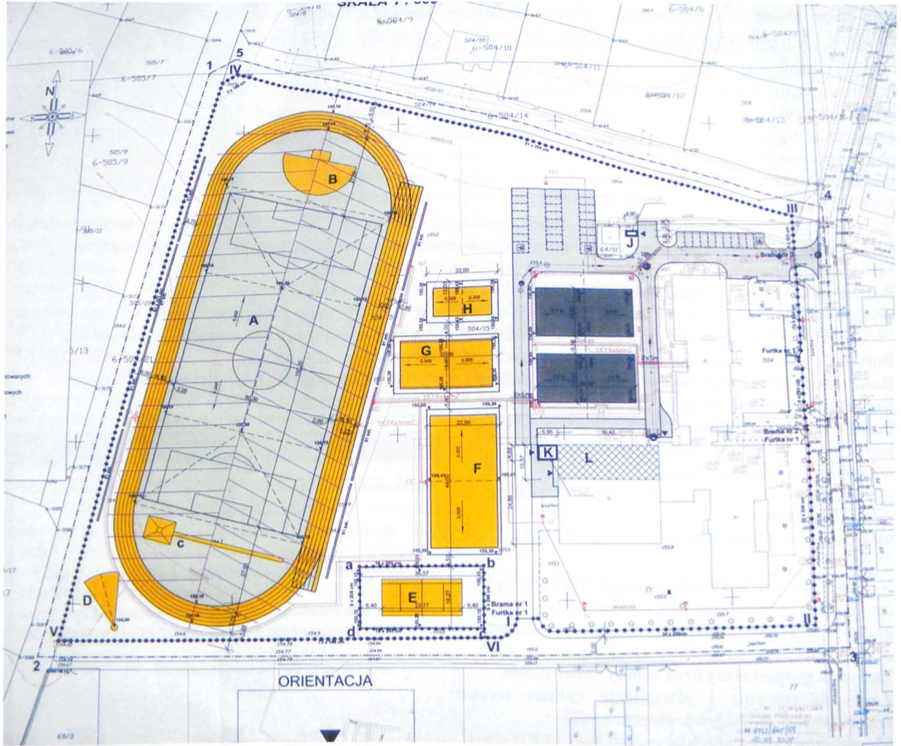
Plan zagospodarowania terenu
