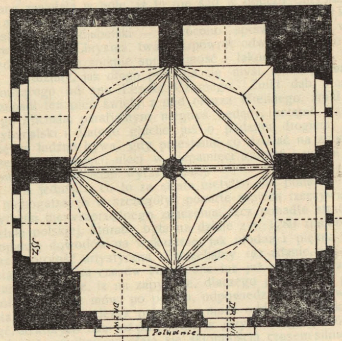
RYS. 1. Wzór pierwotny założenia dośrodkowego, jednostłupowego , w sztuce średniowiecznej polskiej bardzo ulubionego i rozpowszechnionego. Dla wytłumaczenia, skąd pochodzić może układ murów kościoła św. Michała w Lublinie, niesłychanie ciekawego, należy przyjąć koniecznie rozwój rzutu poziomego tak zwany dośrodkowy , to znaczy, oparty na kole wpisanem, jakie tu widzimy zaznaczone linią wykresowaną. Wedle dwudziału całej sztuki polskiej, a przede wszystkim stylu nadwiślańskiego , wypadają po bokach czwartaka czyli kwadratu w osi pionowej i w osi poziomej razem 4 filary, jako przypory. Sklepienie na słupie środkowym jest ośmiopółowe, ma żebra osiowe i żebra ukośne. W polu każdem 3 tarczki, zatem jest to sklepienie polskie, piastowskie , 24 tarczkowe.
