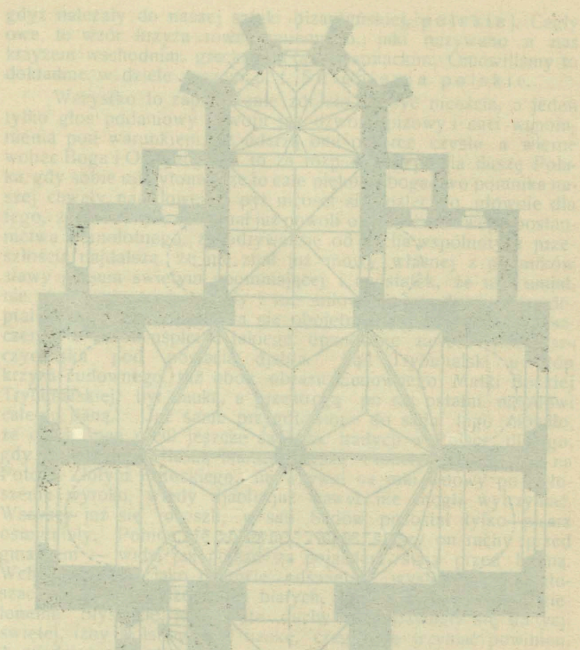
RYS. 2. Rzut poziomy kościoła ś-go Michała w Lublinie, przypuszczalnie od- tworzony na podstawie obrazów i opisów. Układ opiera się o założenie rów- nież dośrodkowe, wychodzące z koła opisanego, jakie daje sześć węzłów sześcioboku wpisanego. Powstaje sposobem takim prostokąt, długość swoją mający w szerokości kościoła. Sklepienie na słupie sześciogrannym, raczej na filarze oparte, ma żebra oddające kształt sześcioboku z przekątnymi. Jest to zatem sklepienie polskie, piastowskie 10 połowe, a gdy w polu każ- dem mamy po 3 tarczki, powstaje sklepienie 30 tarczkowe. Po ręce lewej i prawej mamy po dwie kaplice, przedzielone przyporą. W głębi świątyni część kapłańska po za łukiem tęczowym. Absyda pięcioma bokami ośmiobo- ku zamknięta. Na przedzie wieża. Rysunek służy do wykazania osobliwości wielce niezwyklej w osiągnięciu kościoła o nawie na poprzek wprowadzonej. Wyobrażenie przybliżone.
