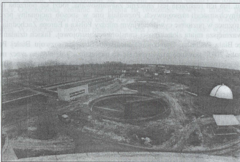
Przebudowa białskiej oczyszczalni ścieków
