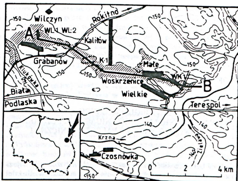
Fig. 1. Zasięg kopalnego zbiornika jeziornego (linie skośne) według Bińki i Nitychoruka z zaznaczonym przebiegiem osi zbiornika A-B i położeniem analizowanych profili osadów jeziornych w Wilczynie – (WL-1, WL-2), Woskrzenicach – (WK-1), Kalitowie – (K-1).
