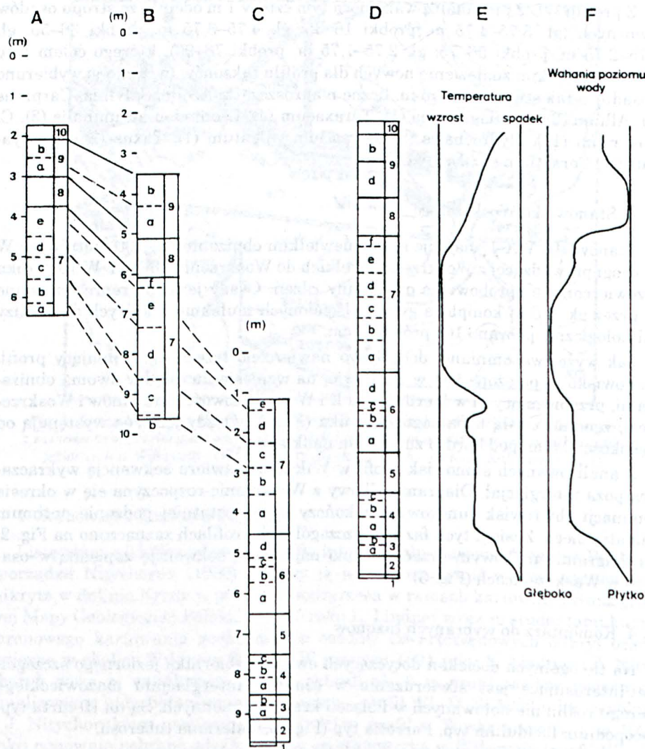
Fig. 2. Korelacja poziomów pyłkowych wyróżnionych w profilach: A – Wilczyn, B – Kaliów, C – Woskrzenice, D – syntetyczny rdzeń zbiorczy z zaznaczonymi poziomami i podpoziomami pyłkowymi.
