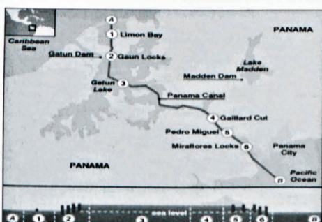
Rys. 7. Mapa Kanału Panamskiego i jego profil pionowy
